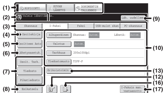
Internet-faksitilan perusnäyttö
